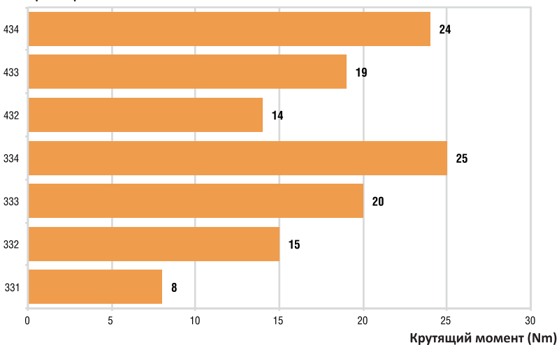
Типоразмер ZL
